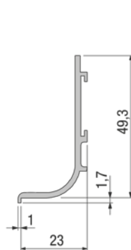
L-Profil
