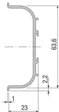
C-Profil
